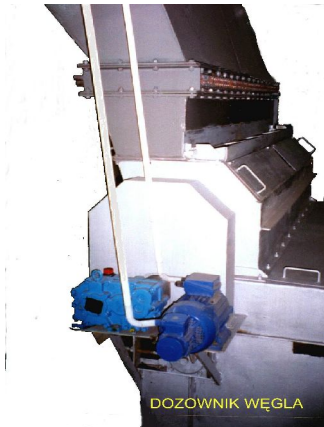
Rys. 2. Bębnowy dozownik węgla
